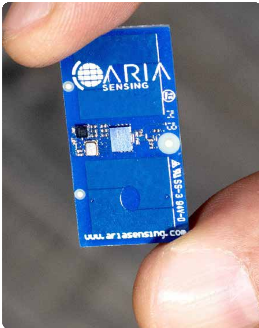
Il modulo radar LT1030EM, il più piccolo modulo radar UWB SMD per applicazioni indoor
